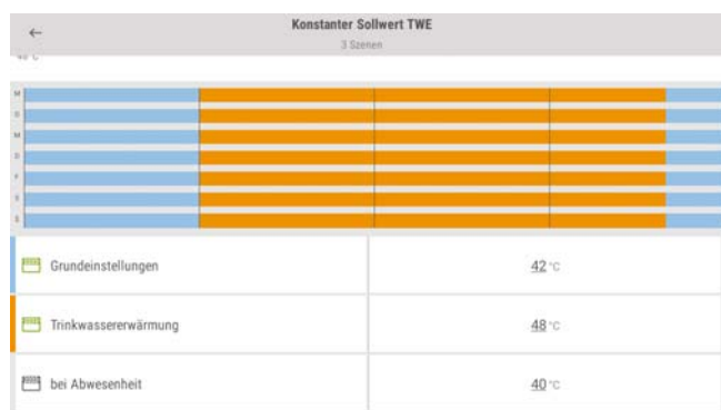
Abb. 4: Zeitprogramm
