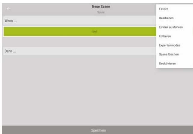
Abb. 26: Neue Szene
